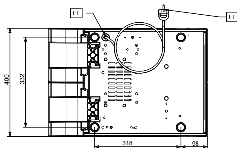
Boven aanzicht
